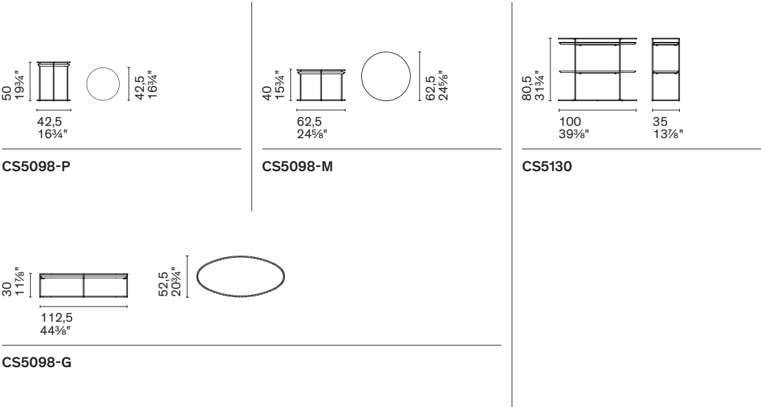
Atollo Tavolino /Coffee table CS5098-G P175 / P18C
